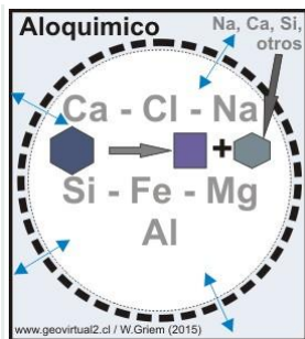
Aloquímico: Sistema abierto, metasomatosis
