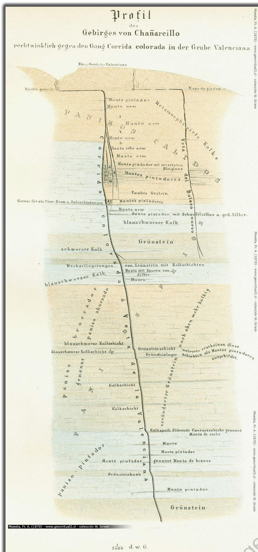
Fig. 2: Profil der Lagerstätte Corrida Colorada
