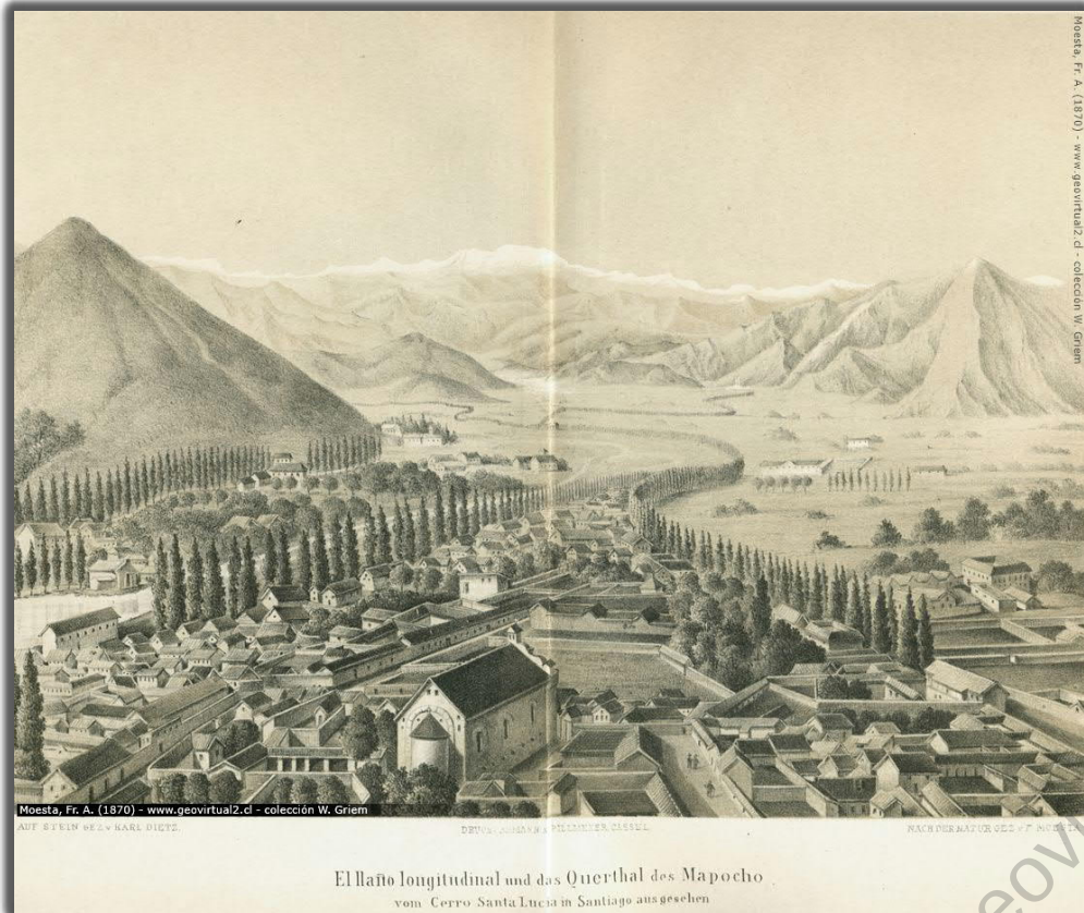
Fig. 4: El Llano longitudinal und das Quertal des Mapocho
